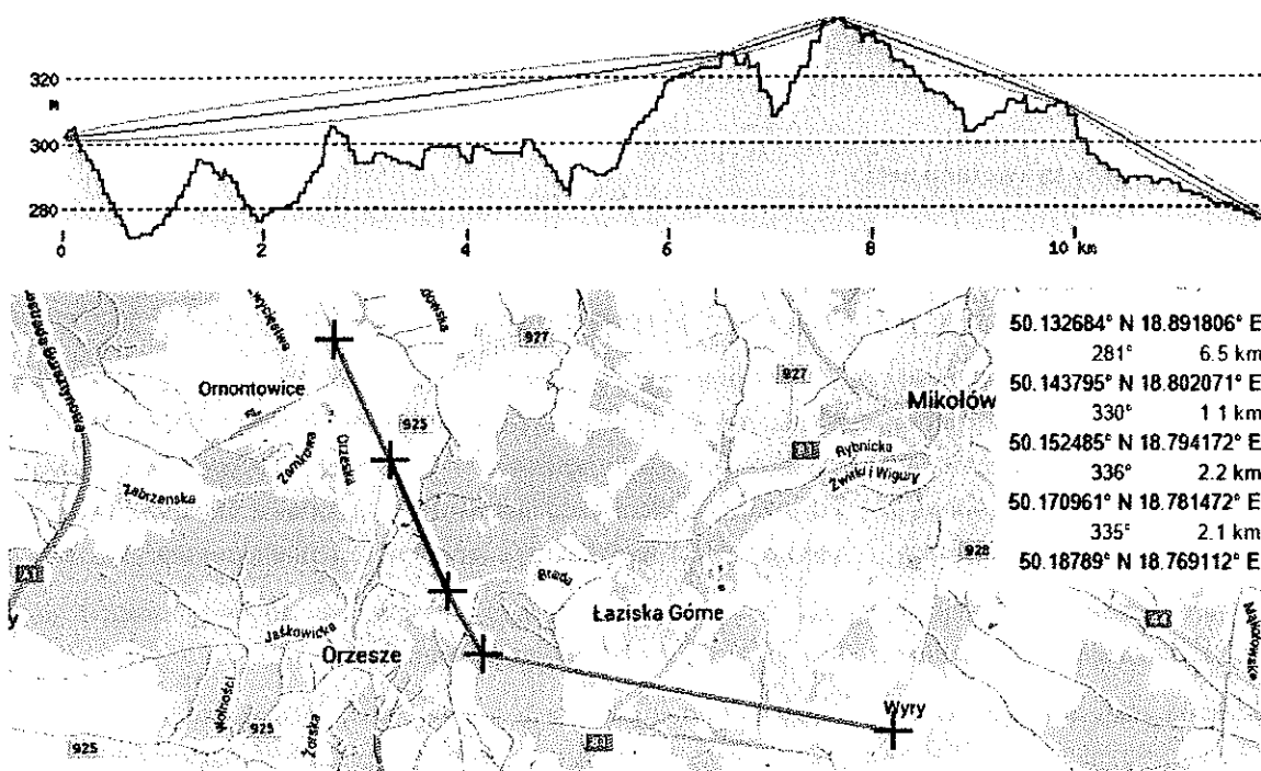
Rysunek 42. Strefy Fresnela zaznaczone na profilu topograficznym przy częstotliwości 24 GHz, krzyżyki na mapie oznaczają umiejscowienie masztów.
