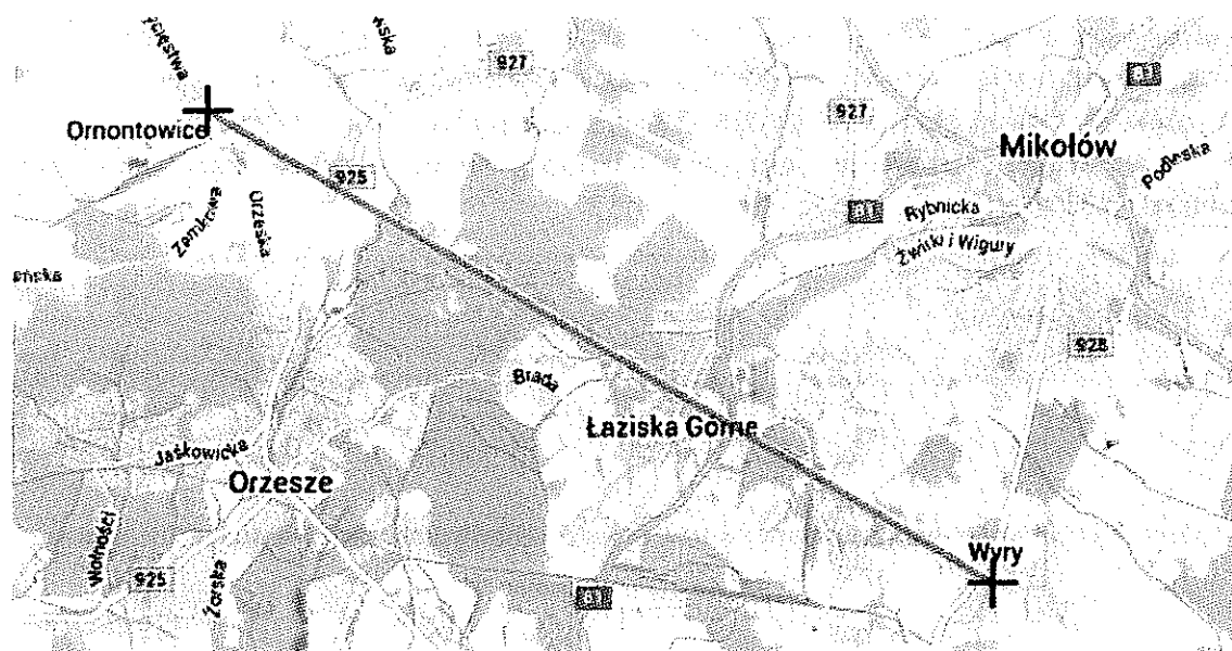
Rysunek 41. Odległość w linii prostej między siedzibami Gmin Ornontowice i Wiry, źródło: http://www.heywhatsthat.com/profiler.html
