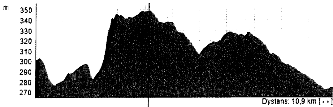
Rysunek 40. Profil topograficzny Ornontowice – Wyry, zaznaczono najwyższy położony punkt między gminami (okolicie Łazisk Górnych)
